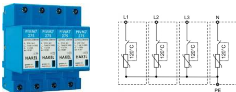
Obr. 4 – SPD 4+0 a schéma vnitřního zapojení
