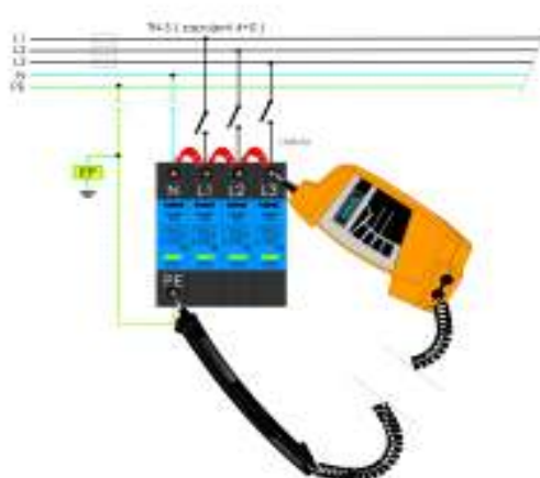
Obr. 5 – Měření SPD 4+0
