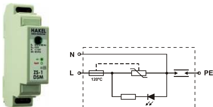
Obr. 7 – Jednofázová SPD s LED indikátorem
