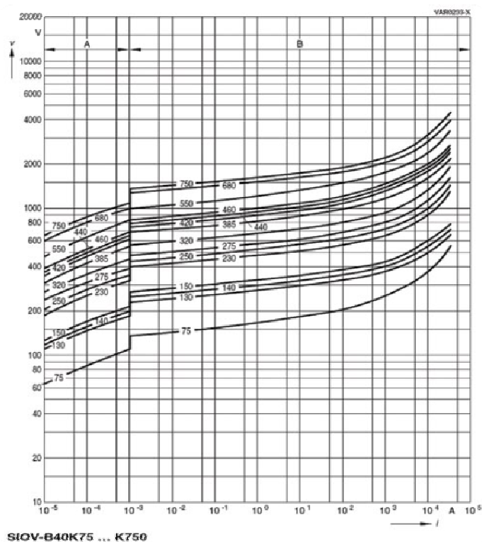
Obr. 3 – Miliampérové body rôznych typů varistorů
