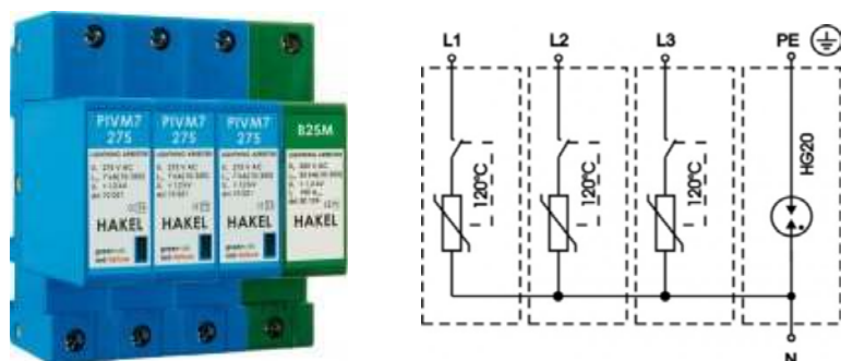
Obr. 5 – SPD 3+1 a schéma vnitřního zapojení
